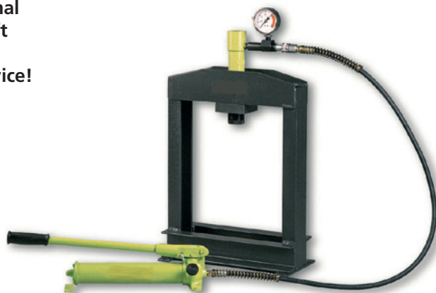
Tischpresse mit starrem Rahmen und Handpumpe
